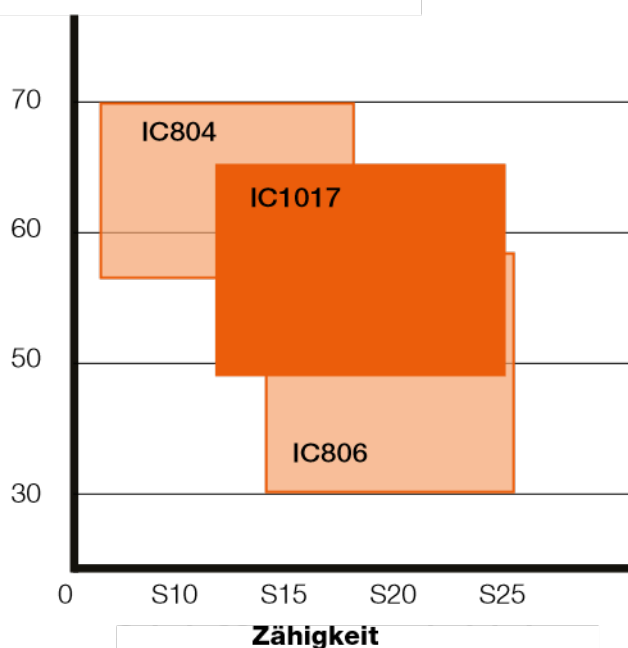
Schnittgeschwindigkeit
